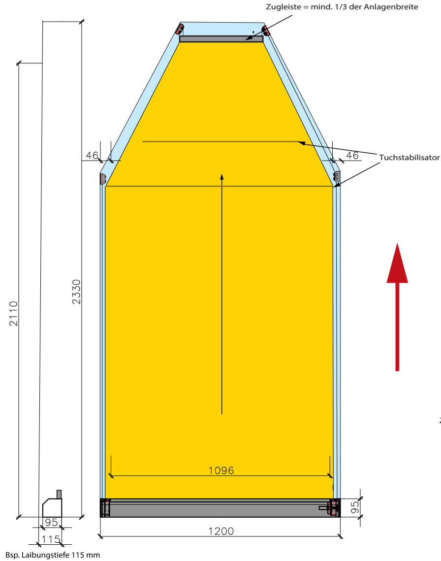
Bsp. ausgefahrenes Innenrollo für Giebfenster UNO 95.2 am Mustermaß Breite 1200 x Höhe 2330 mm
