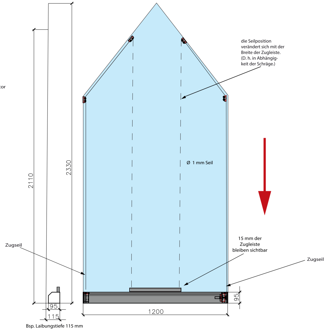
Bsp. eingefahrenes Innenrollo für Giebelfenster UNO 95.2 am Mustermaß Breite 1200 x Höhe 2330 mm
