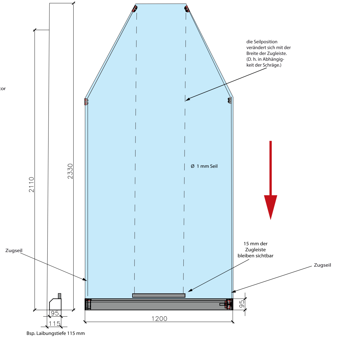
Bsp. eingefahrenes Innenrollo für Giebfenster UNO 95.2 am Mustermaß Breite 1200 x Höhe 2330 mm
