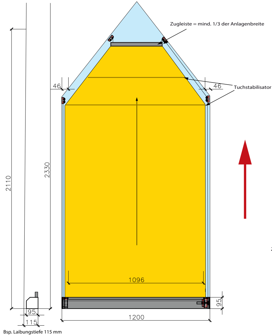
Bsp. ausgefahrenes Innenrollo für Giebelfenster UNO 95.2 am Mustermaß Breite 1200 x Höhe 2330 mm
